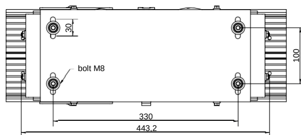
Опорный кронштейн РСТ7-MB125 для токосъемной тележки
