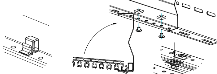
Защелка PR7-MCB в нижней части опорного профиля SP7
